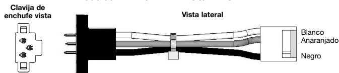
Diagrama del enchufe de adaptador (ADK) para los modelos KIDDE/FYRNETICS/LIFESAVER®:
